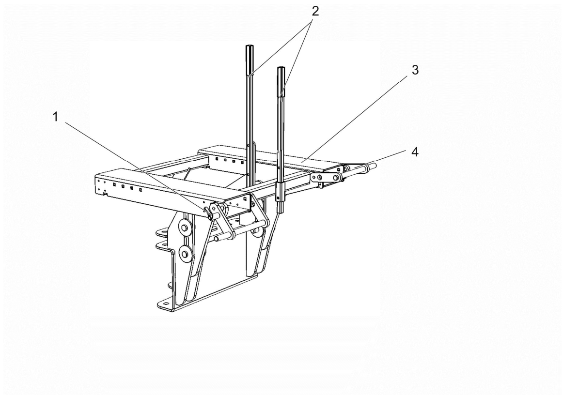
Abbildung 7 Gabelzinkenaufnahme
