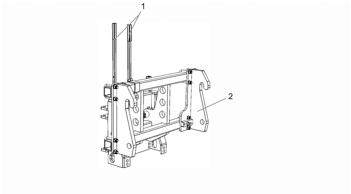
Abbildung 8 Radladeraufnahme
