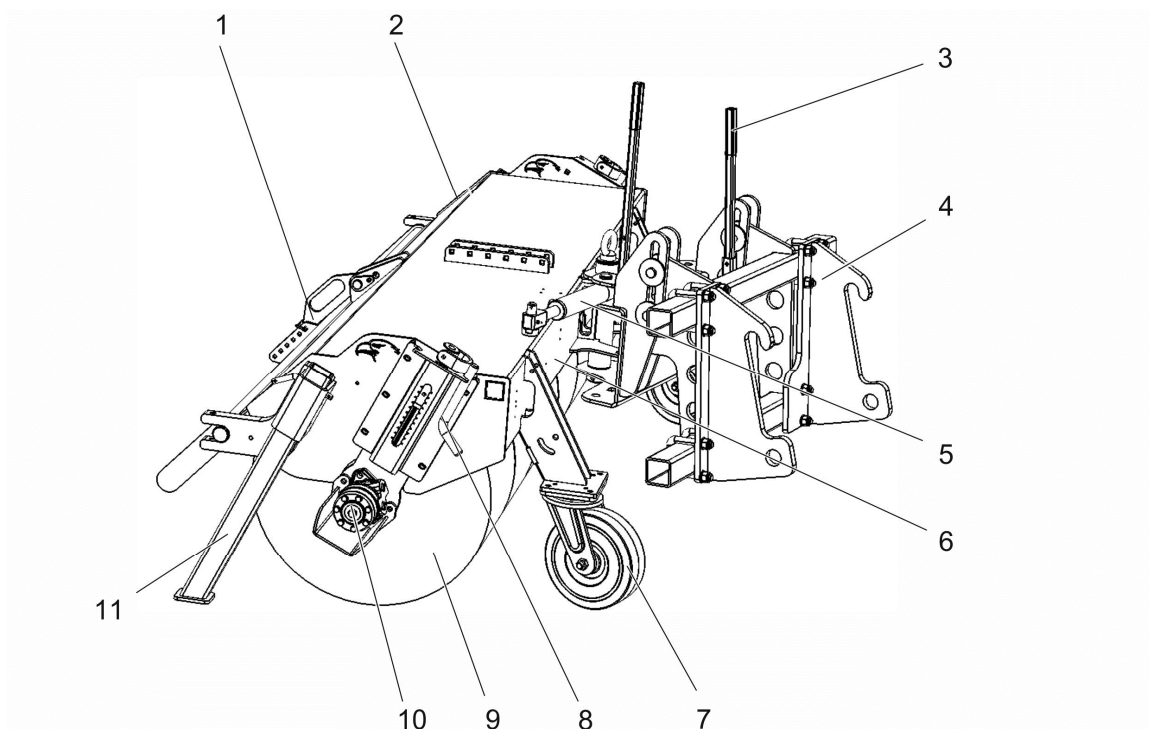
Abbildung 2 Kehmaschine K 600
