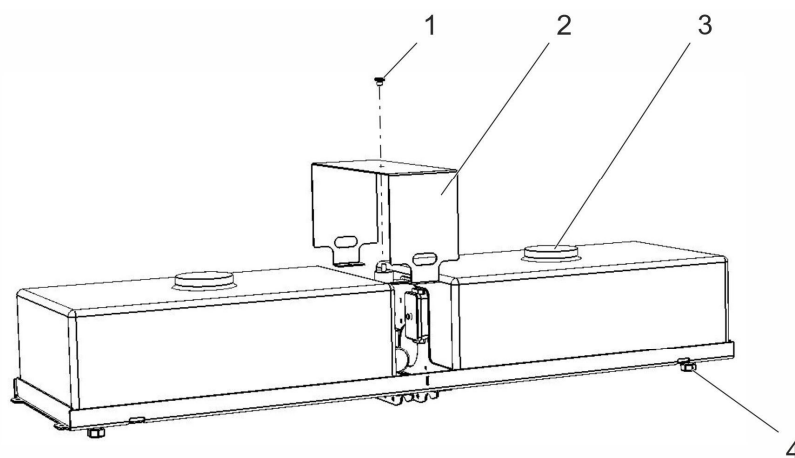
Abbildung 9 Wassertank 240 Liter
