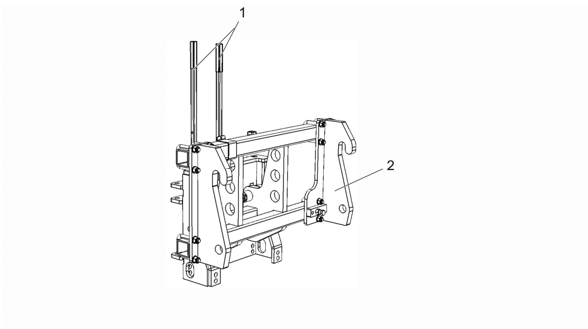
Abbildung 4 Anbausystem mit Peilstäben
