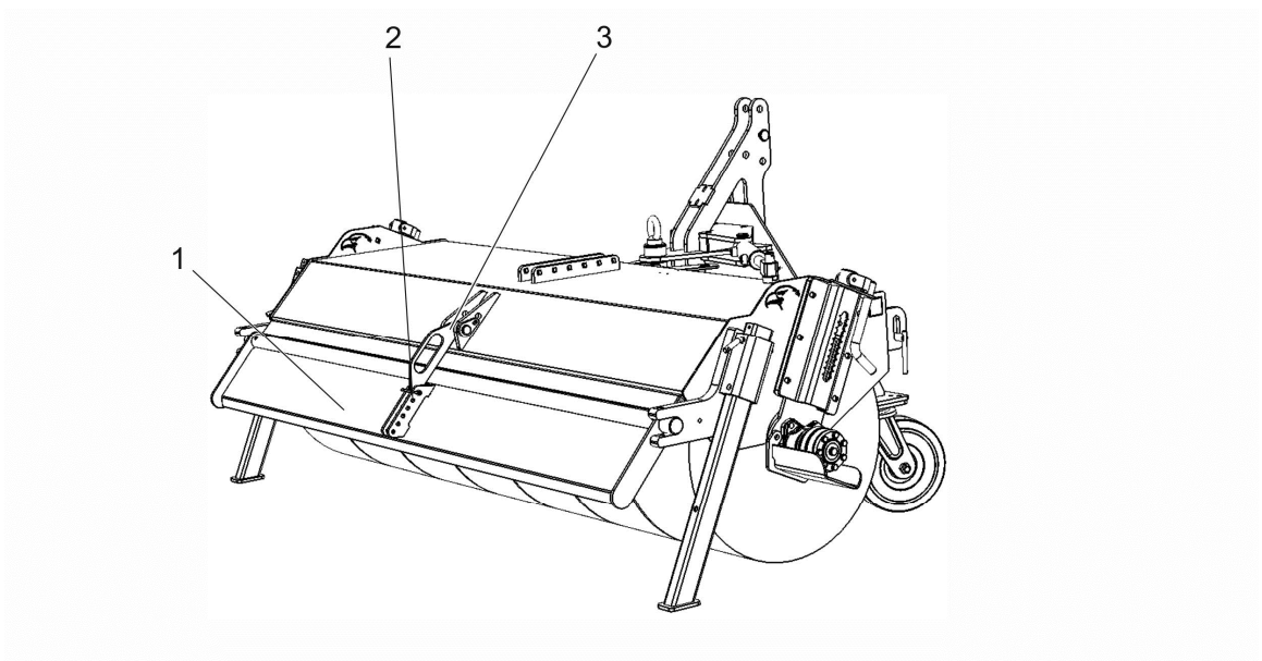
Abbildung 11 Verstellung Spritzschutzblech
