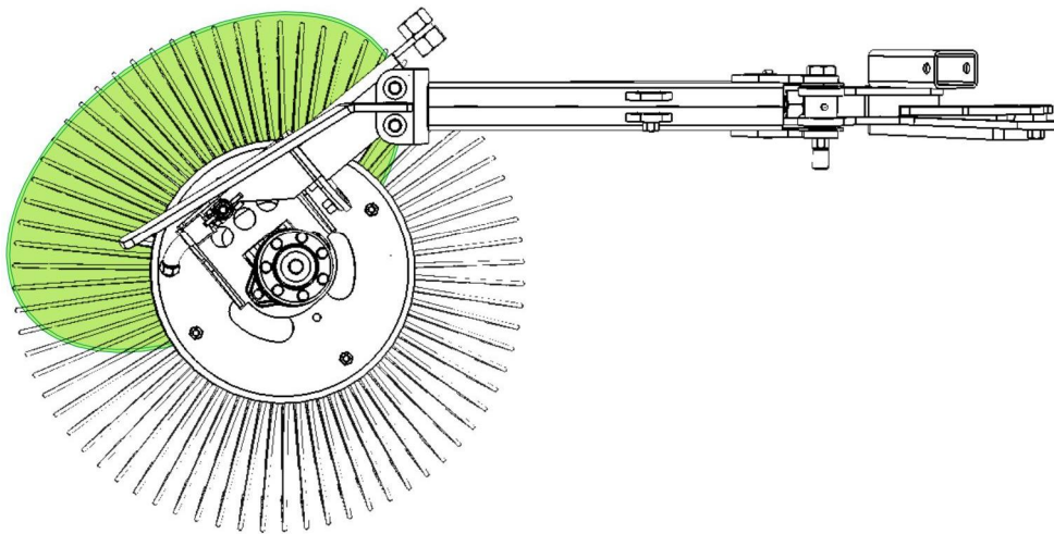
Abbildung 18 Eingriff Seitenkehrbesen
