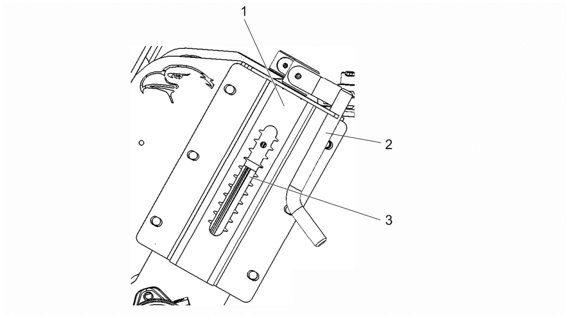
Abbildung 15 Höhenverstellung Kehrwalze
